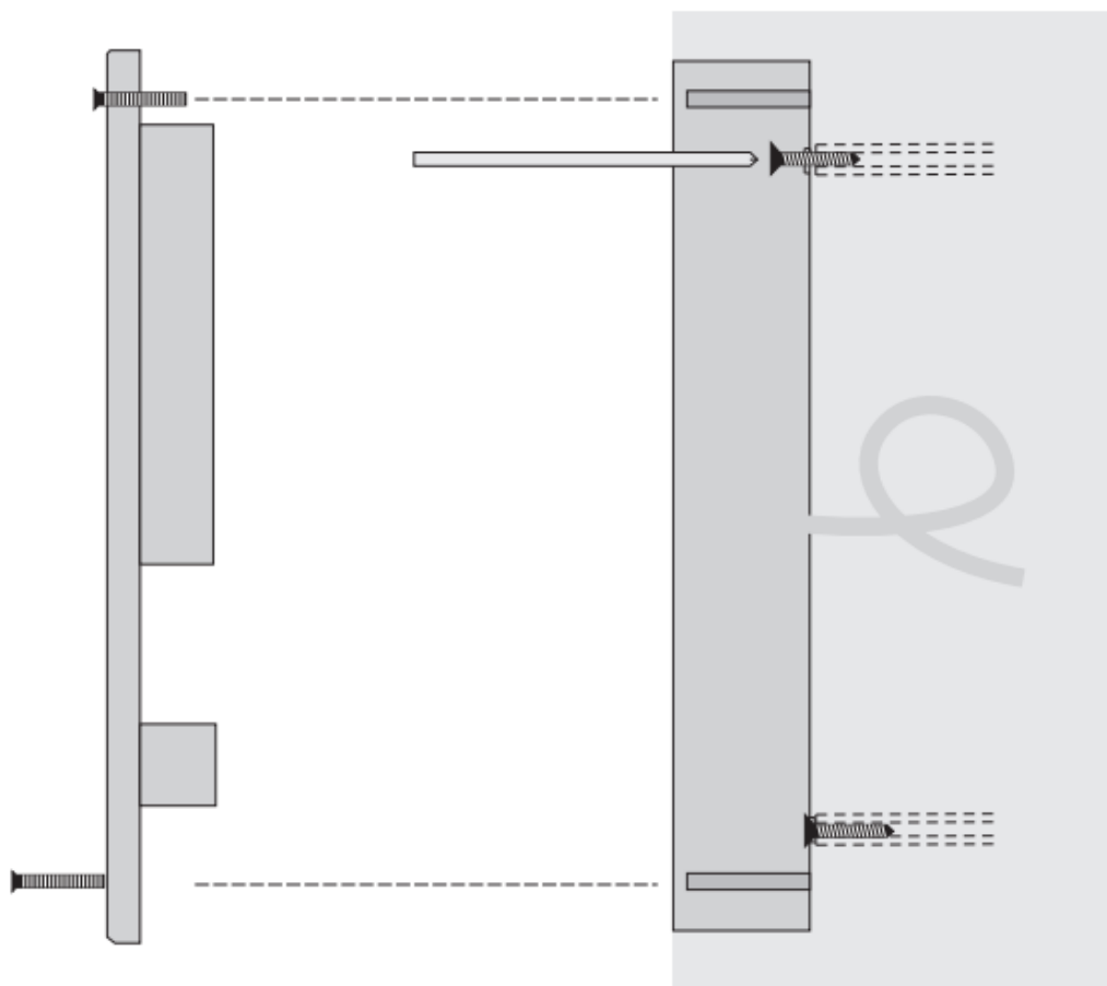
Рисунок 3 – Врезной монтаж устройства
